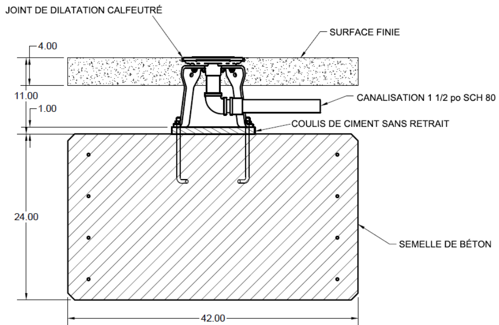
DÉTAIL DE LA BASE PLAYPHASE
