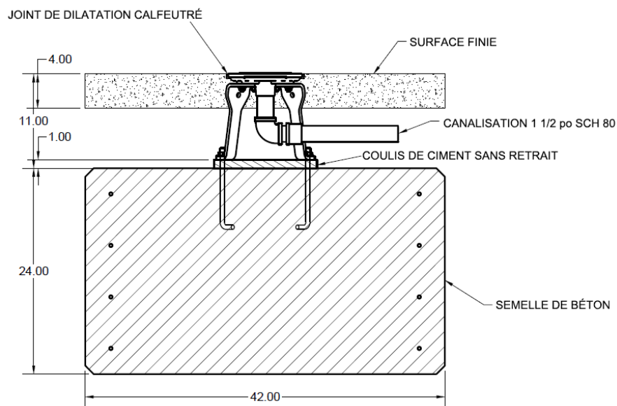
DÉTAIL DE LA BASE PLAYPHASE
